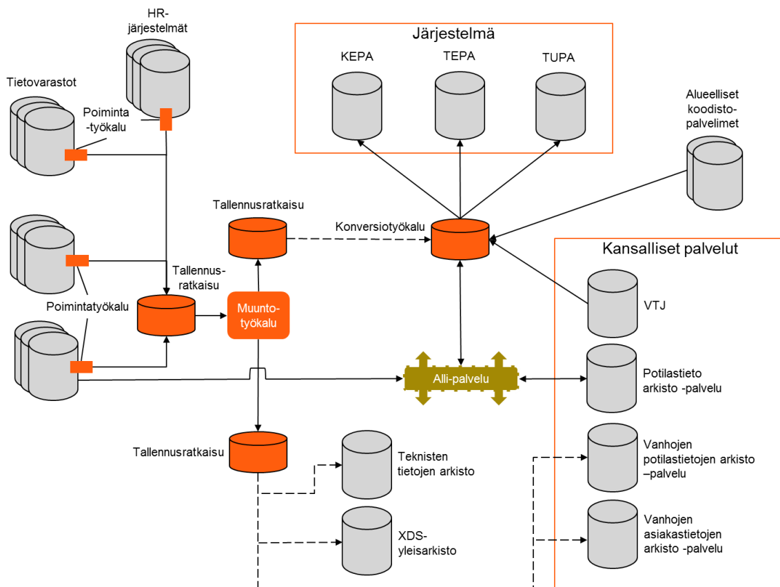
Kuva 2. Teknisen arkkitehtuurin yleiskuva
