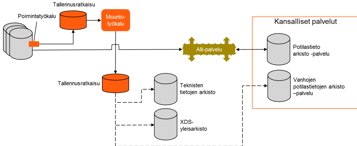
Kuva 4. Terveysthuollon arkistoinnin tekninen arkkitehtuuri
