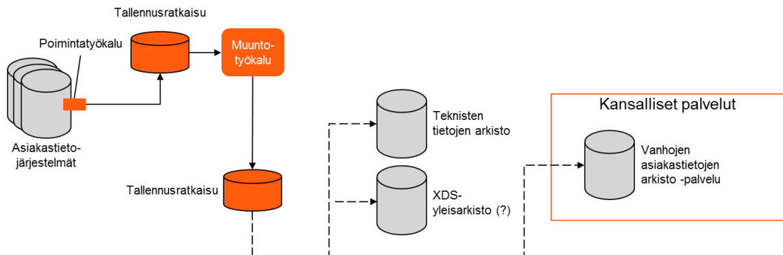
Kuva 6. Sosiaalihuollonhuollon arkistoinnin tekninen arkkitehtuuri
