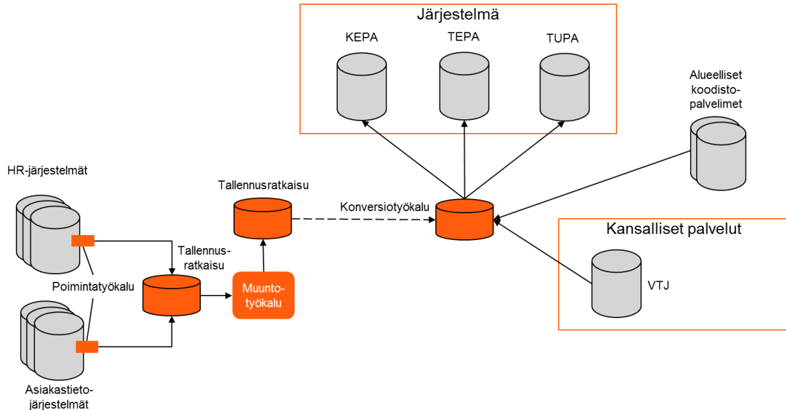
Kuva 5. Sosiaalihuollon Järjestelmään tehtävien tiedonsiirtojen tekninen arkkitehtuuri
